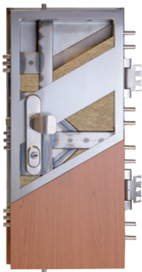
Rez dverí RAD ELITE
