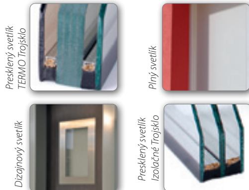
Dvere s bočným svetlíkom a nadsvetlíkom
