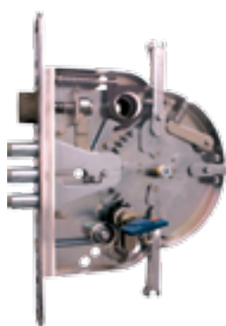
Trezorový rozvorový mechanizmus ADLO RESIST MT RAD ELITE //
