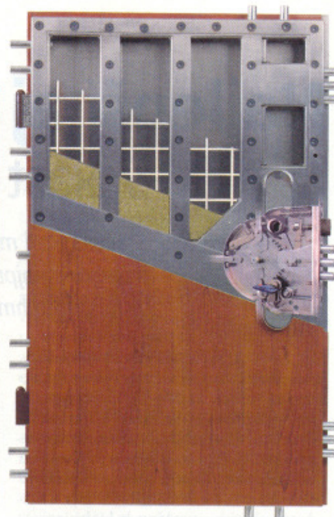
Konštrukcia dvojitých bezpečnostných dverí s výstuhami, bezpečnostným zámkom, izoláciou, povrchovou úpravou, pevnými (vľavo) a pohyblivými (vpravo, dole, hore) istiacimi bodmi (ADLO – Bezpečnostné dvere)
